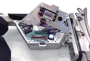
エレクトロニックトリガー機関部
